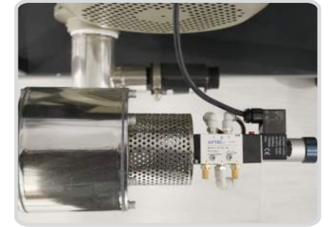
Vakum Kesme Valfi
